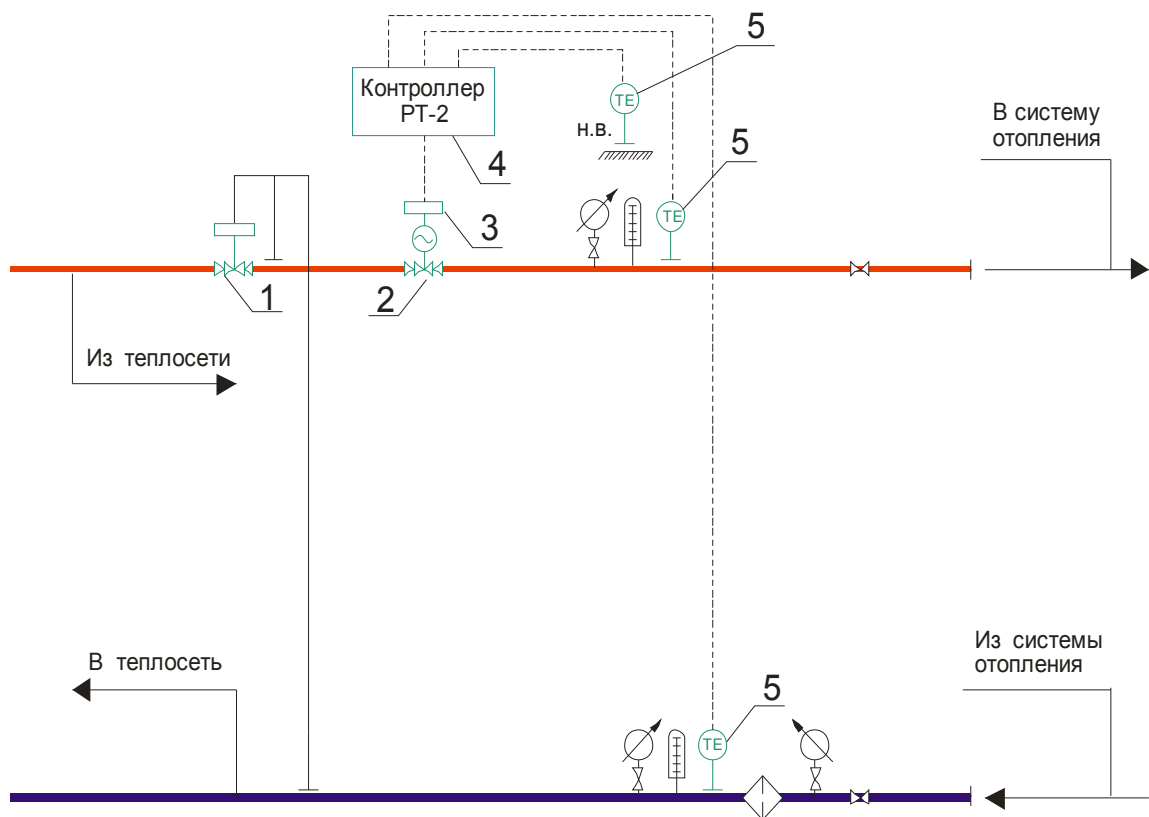
Рисунок П 3.5. Принципиальная гидравлическая схема узла регулирования для системы ОТП.
