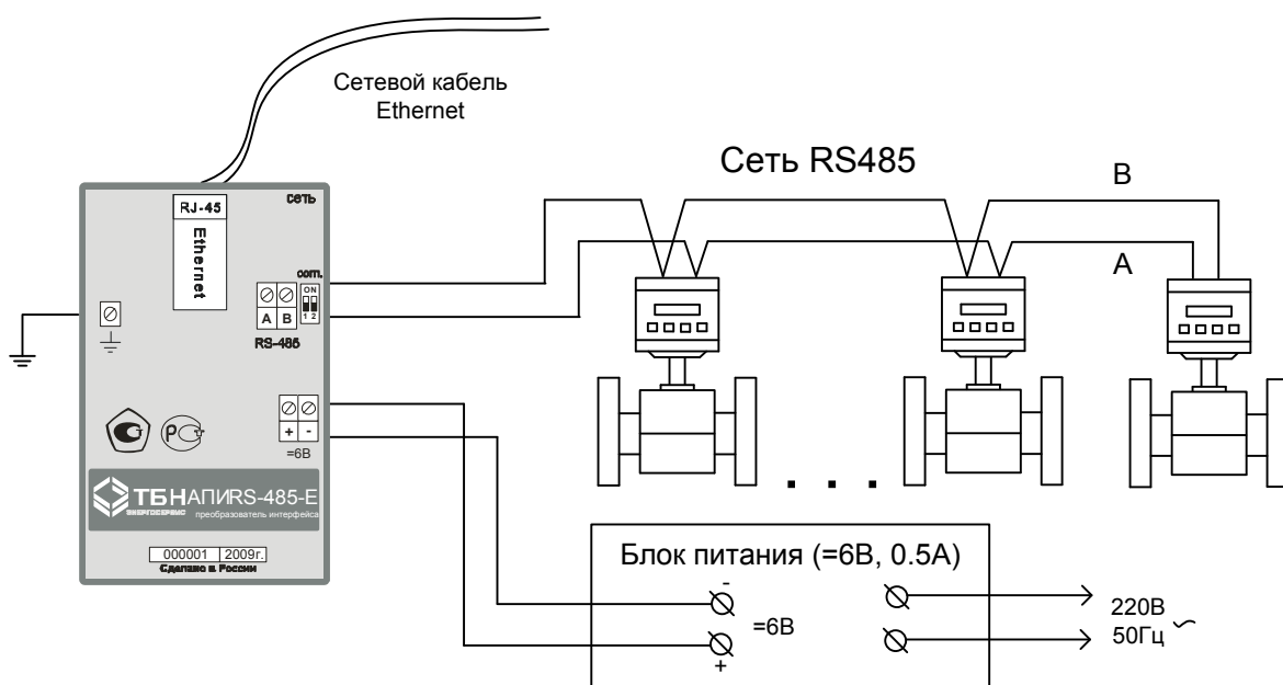
Рисунок П1.2. Альтернативная схема монтажа электрических цепей. Применяется в исключительных случаях под ответственность заказчика без использования МГЗ из комплекта поставки адаптера. Данная схема допустима только при гарантированной гроозащищенности точки доступа в сеть Ethernet.
