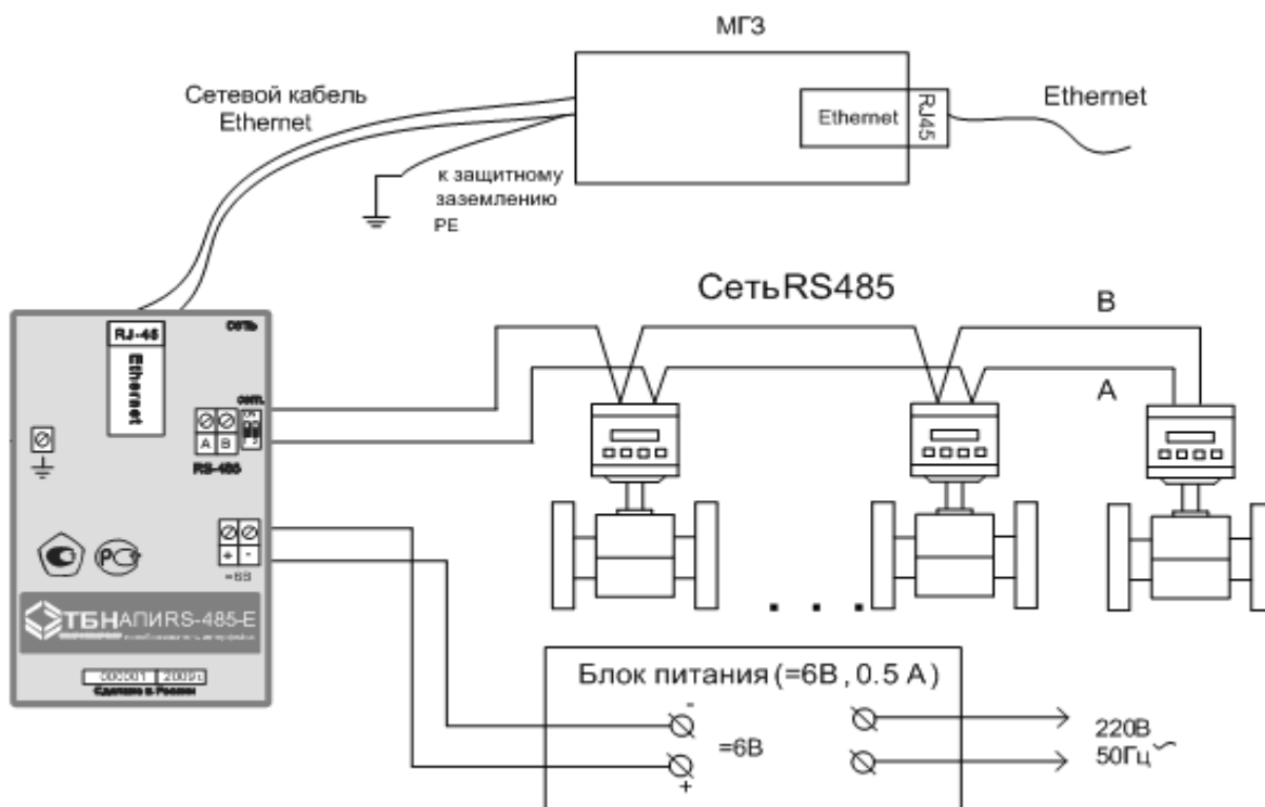
Рисунок П1.1. Схема монтажа электрических цепей. Использование модуля гроозащиты обязательно!
