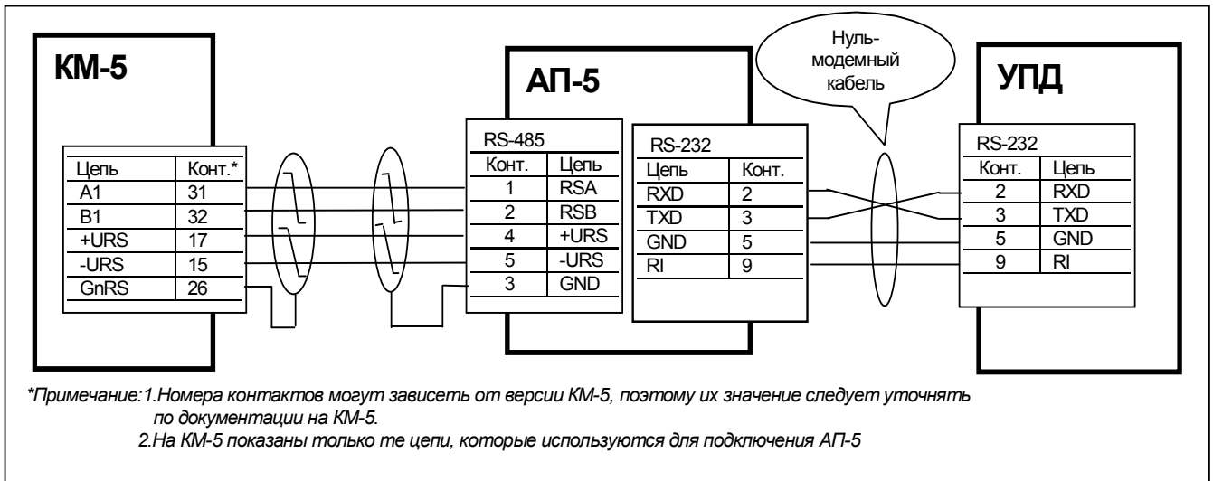
Рисунок 3 — Схема монтажа для подключения через адаптер периферии АП-5
